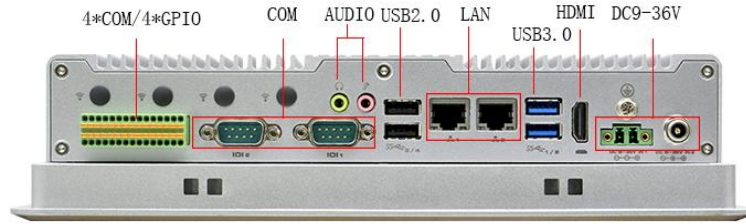
底部I/O视图
