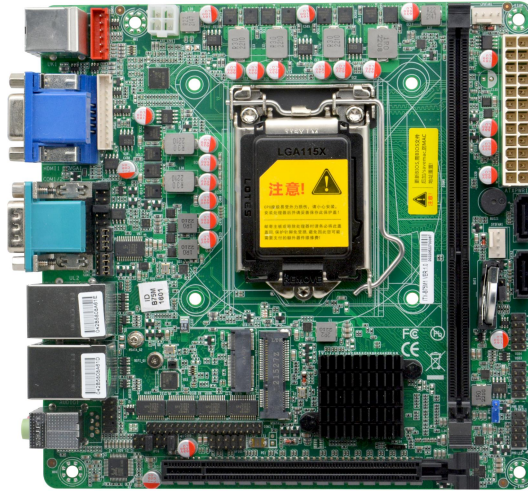
ITX-B75M1 VER:1.0 正面图
