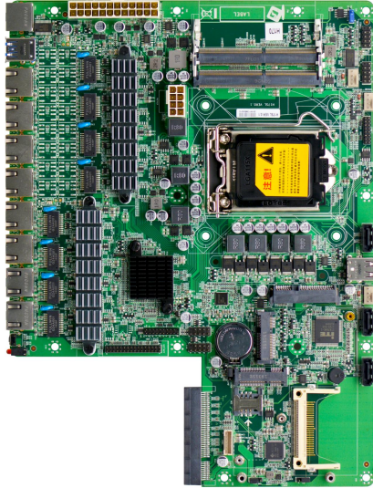
H17SL VER:1.0 板正面图
