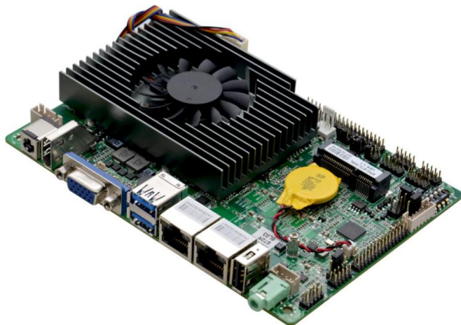
EPIC-E73_I526L VER:1.1 主板侧面图
