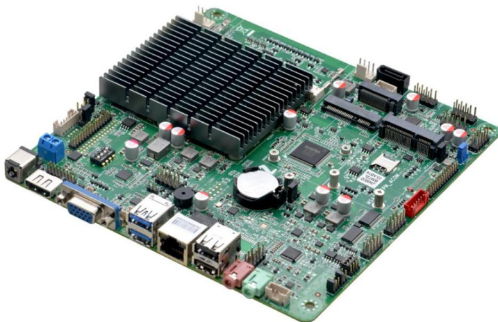
ITX-B347_J112L VER:1.2 主板侧面图
