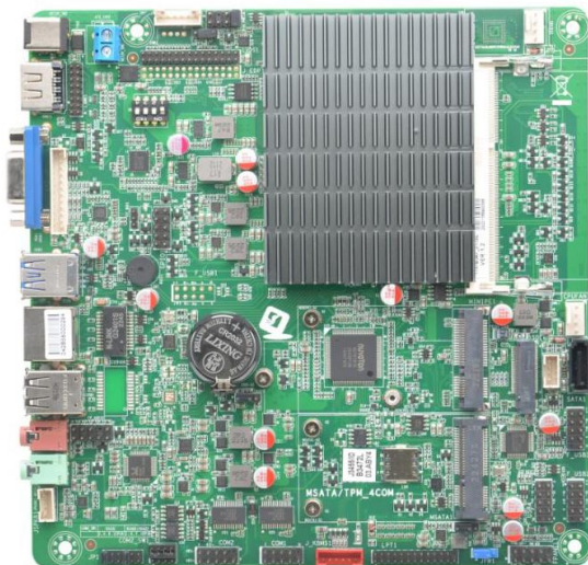
ITX-B347_J112L VER:1.2 主板正面图
